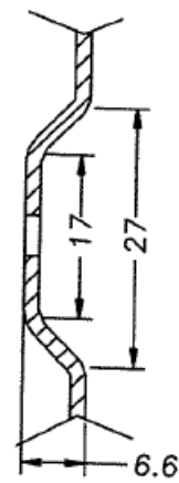
SECTION A-A SCALE: 4:1
