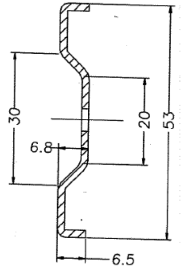
SECTION A-A SCALE: 4:1
